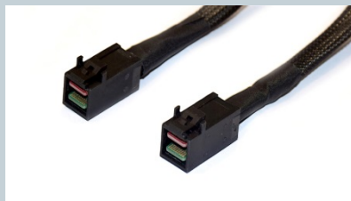
Internal Mini SAS HD SFF-8643 to Mini SAS HD SFF-8643
